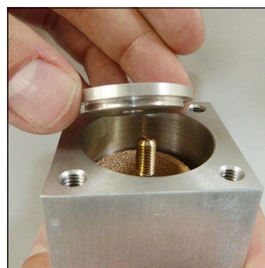
Abb. 5 - Filterscheibe und Unterlegscheibe aufsetzen
