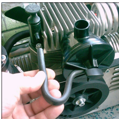
Abb. 1 - Entlüftungsschlauch am Öleinfüllstutzen abziehen
