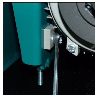
Abb. 1 - Befestigungsschrauben lockern
