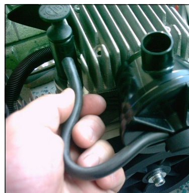
Abb. 6 - Entlüftungsschlauch am Öleinfüllstutzen montieren
