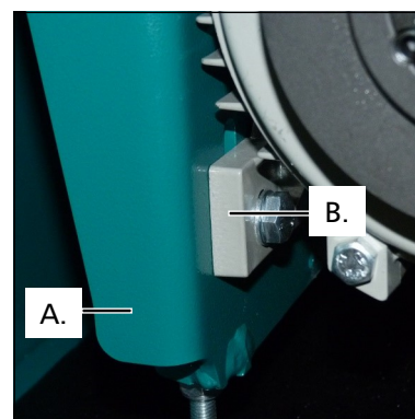
Abb. 4 - Motor und Motorplatte müssen parallel sein
