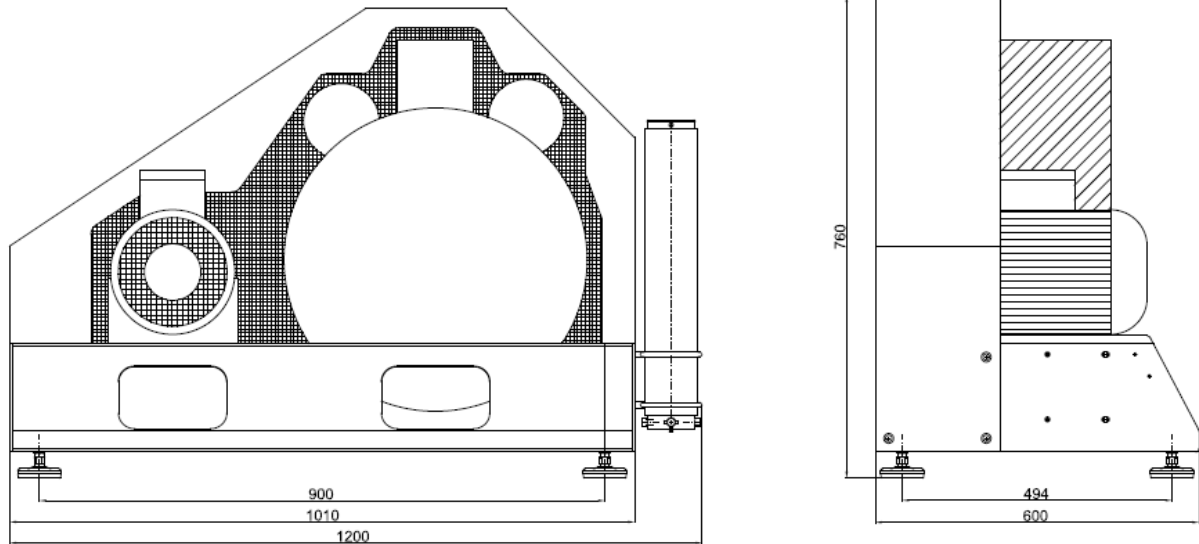
Abb. Einbaumaße
