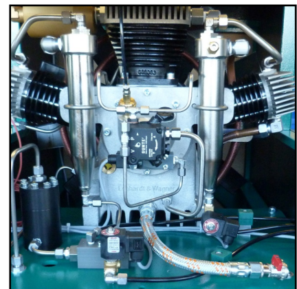
Öl- / Wasserabscheider 1. + 2. Stufe
