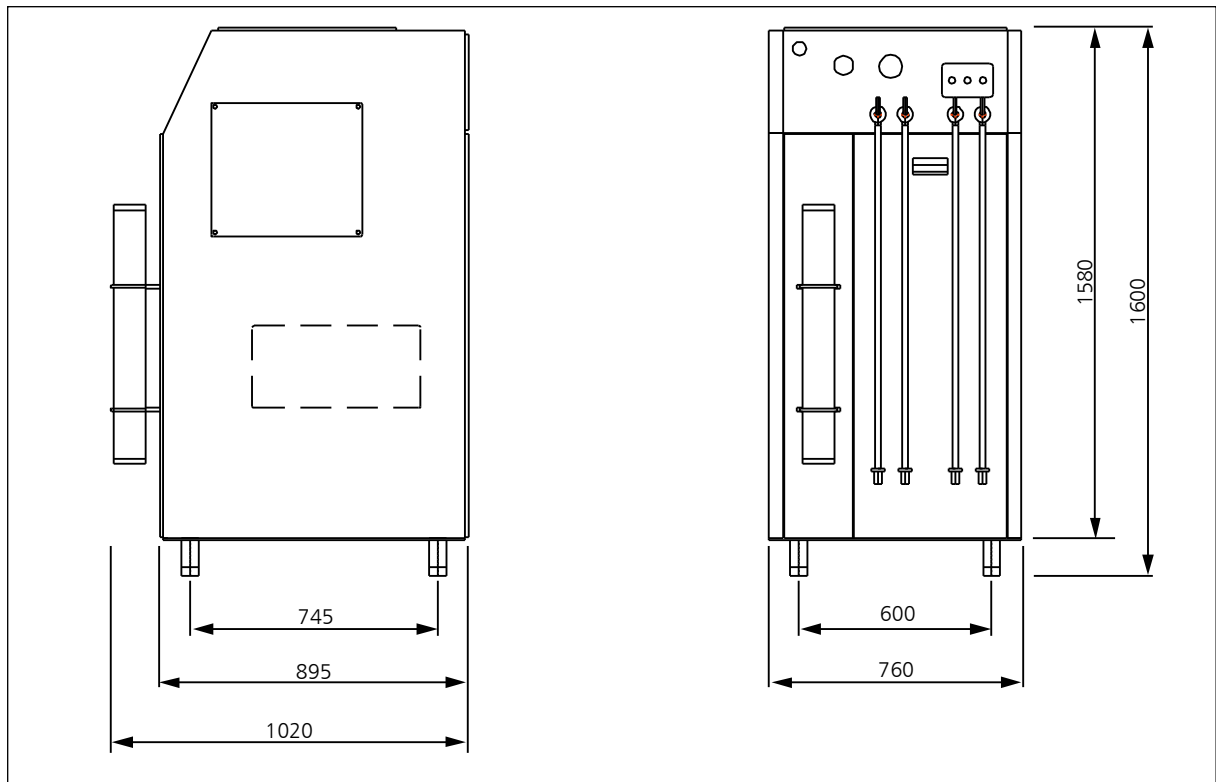
Abb. Einbaumaße
